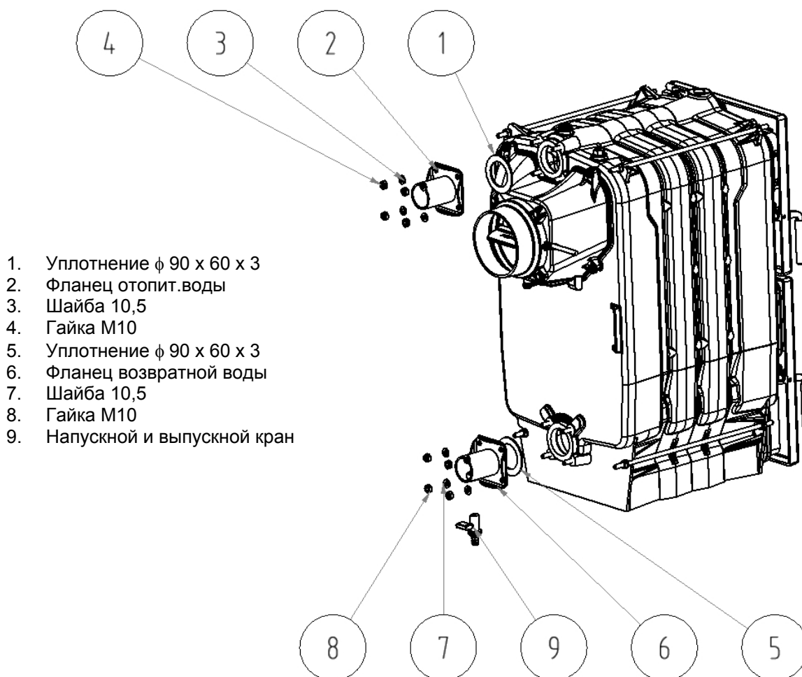
Рис. № 14 Монтаж котельного корпуса
