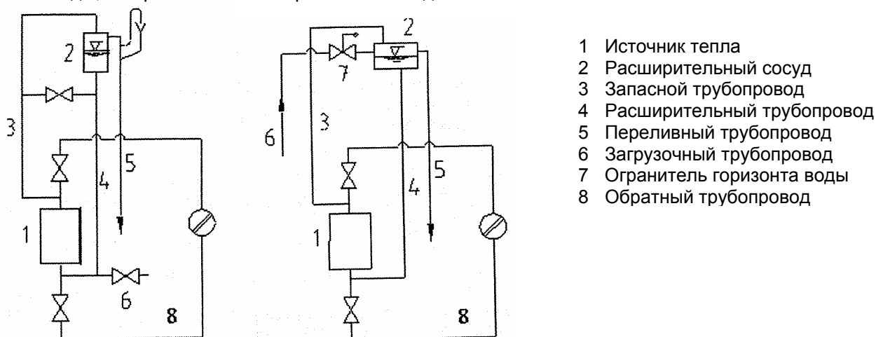
Рис. № 9 Образцы подключения открытых расширительных сосудов
