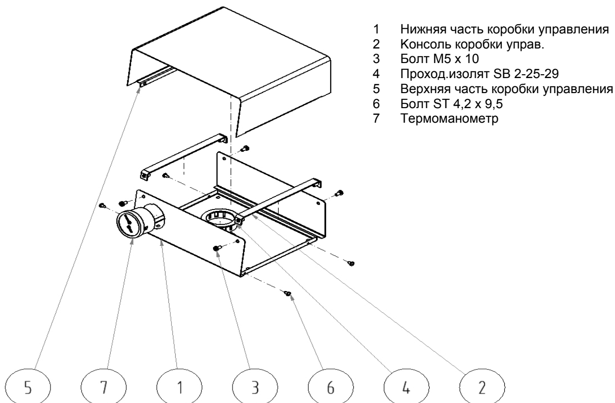
Рис. № 20 Монтаж коробки управления
